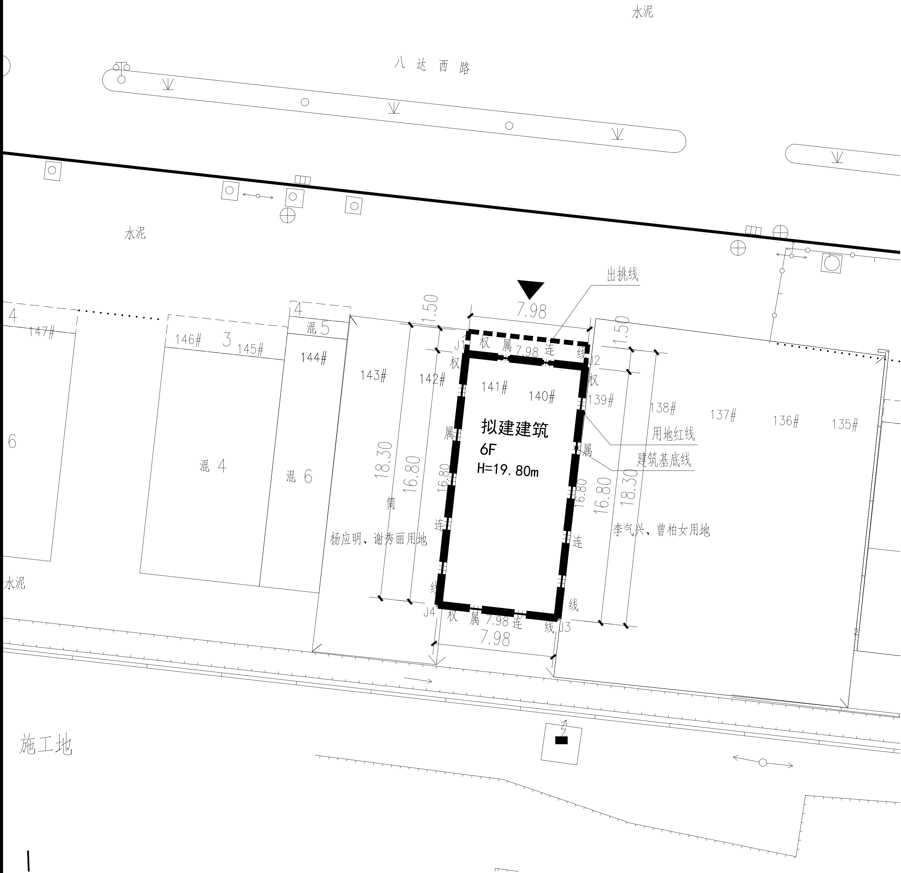
总平面图 1:300
