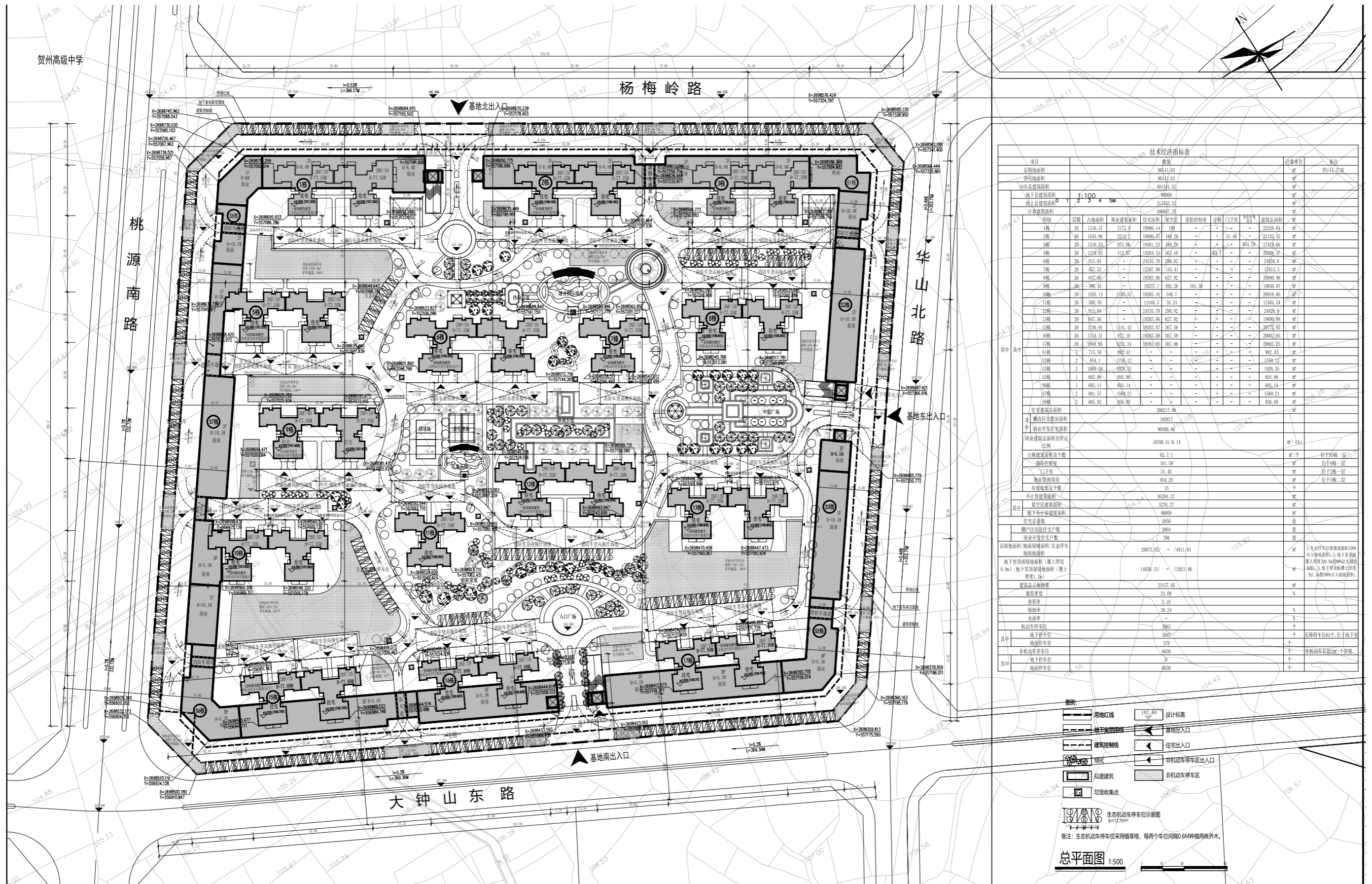
修改前 总平面图
