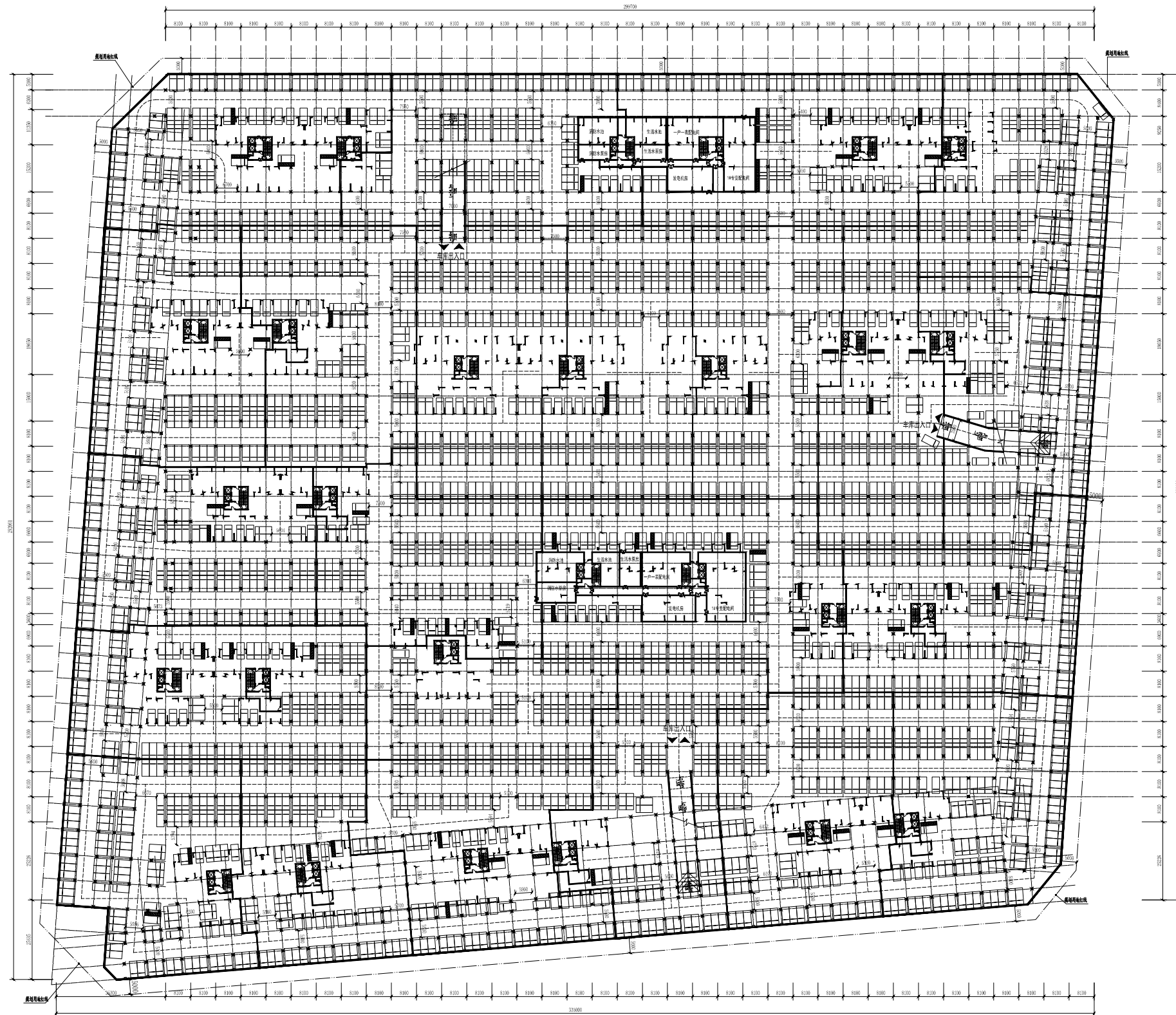
地下室平面图 1:500 地下室建筑面积: 92028平方米 共设置20个防火分区 地下室停车位: 共2483位 (其中普通停车位2421个, 无障碍停车位62个 (占本项目总停车位2%))
